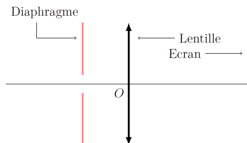
FIGURE 2 – Modélisation optique simplifiée de l'œil humain.
