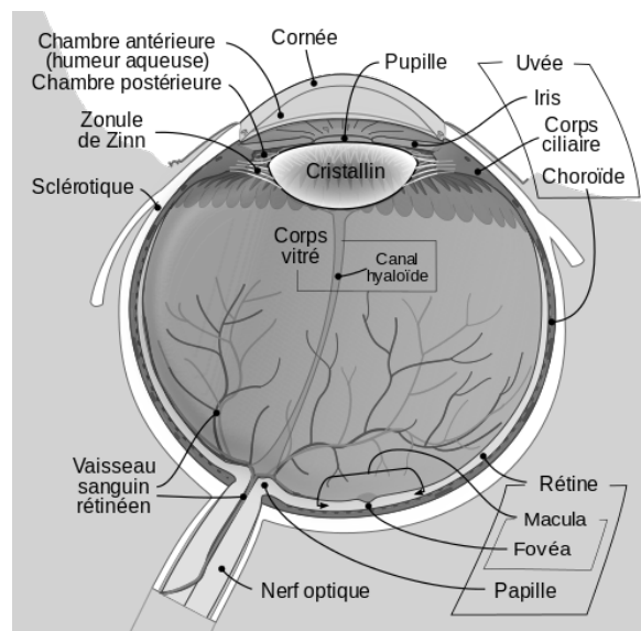
FIGURE 1 – Schéma anatomique d'un œil humain.
