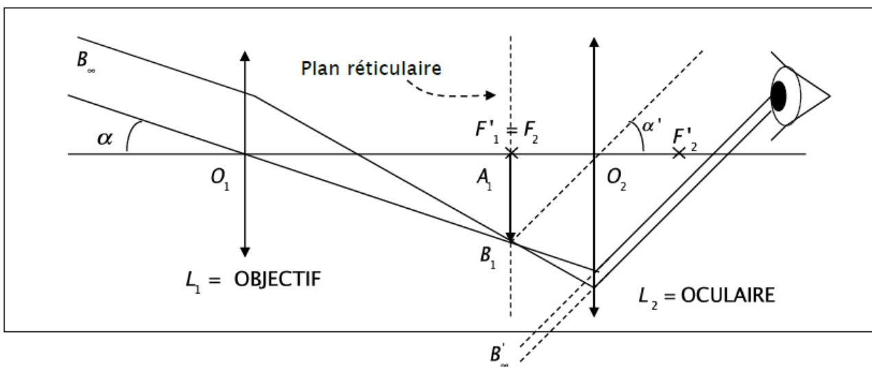
FIGURE 5 – Schéma de principe d'une lunette astronomique.
