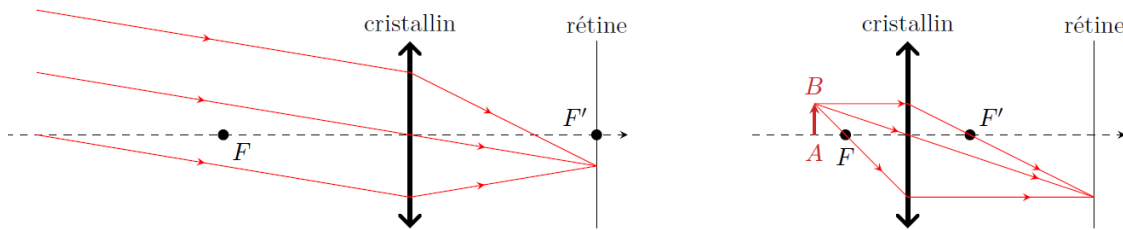
FIGURE 3 – Formation des images vues au punctum remotum à gauche et au punctum proximum à droite.
