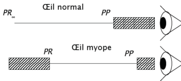
FIGURE 4 – Comparaison des punctum remotum et punctum proximum pour un œil emmétrope et un œil myope
