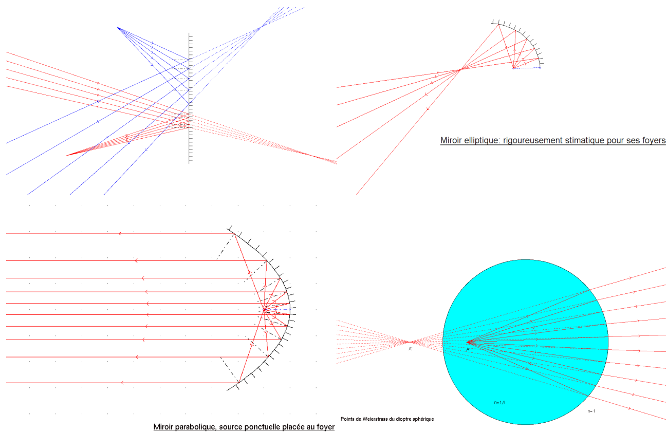
FIGURE 2 – En haut à gauche : miroir plan, stigmatique pour tous les points de l'espace. En haut à droite : miroir elliptique, stigmatique uniquement pour les foyers de l'ellipse (c'est-à-dire un seul couple de points). En bas à gauche : miroir parabolique, stigmatique pour un point à l'infini et le foyer de la parabole (c'est cette propriété qui est utilisée dans la réception de signaux satellitaires via une parabole). En bas à droite : boule sphérique, stigmatique pour un couple de points appelés points de Weierstrass.
