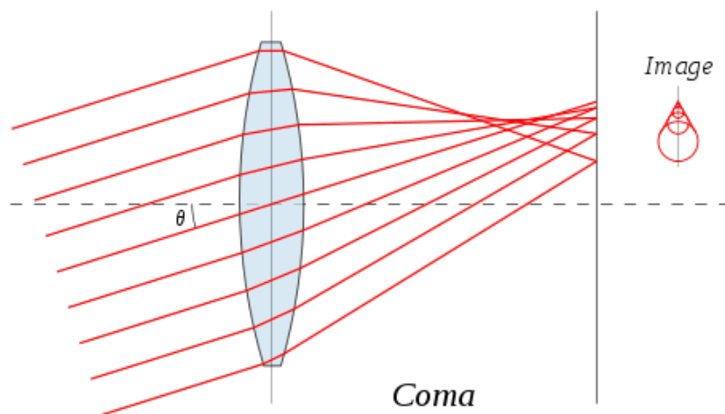
FIGURE 1 – Un exemple d'aberration géométrique pour un système dioptrique : l'aberration de coma. Si le système était parfaitement stigmatique, tous les rayons seraient concourants après le système. Comme le faisceau incident est très incliné, ils se croisent en fait après la lentille en différents points, formant une infinité d'images étalées dans l'espace. Si l'étalement de toutes ces images est plus large que la résolution du détecteur utilisé, l'image sera considérée floue.
